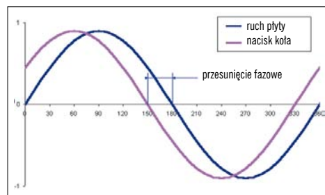
PRZESUNIĘCIE FAZOWE AMPLITUDEY DRGAŃ WYMUSZAJĄCYCH PŁYTĘ TESTERA (KOLOR GRANATOWY) I AMPLITUDEY WYMUSZANYCH DRGAŃ KOŁA (KOLOR RÓŻOWY)
