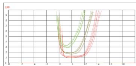
POMIAR WSPÓŁCZYNNIKA CAP URZĄDZENIEM EXPERT BENCH (KOLOR ZIELONY SPRAWNOŚĆ AMORTYZATORA 100%, KOLOR SZARY 50%, KOLOR CZERWONY 20%)
