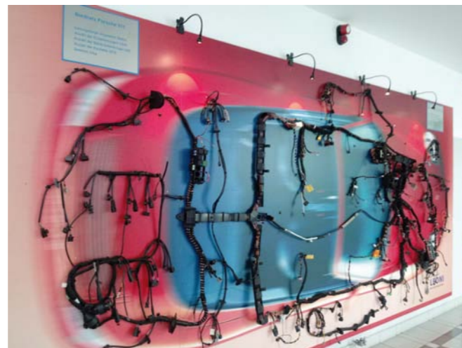
WIĄZKA KABLOWA PORSCHE 911 W SKALI 1:1
